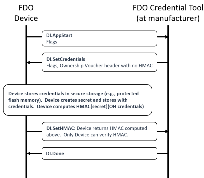
Figure 10 DI Protocol Diagram
